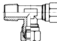
T-kus L, vnější kuželový závit
